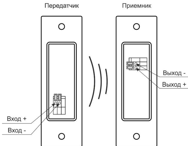
Рис 2. Схема подключения
