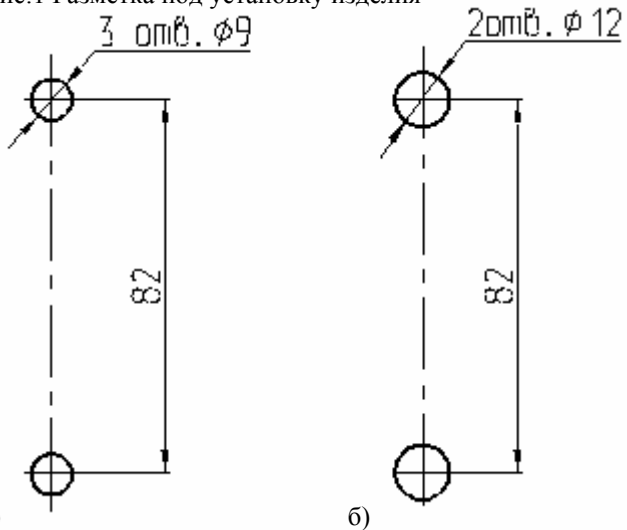
Рис.1 Разметка под установку изделия
