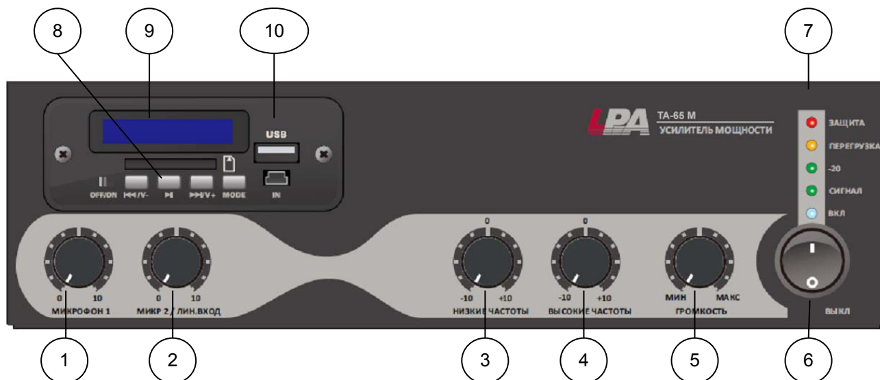
Рис. 3.1. Схема расположения средств управления LPA-TA-65M
