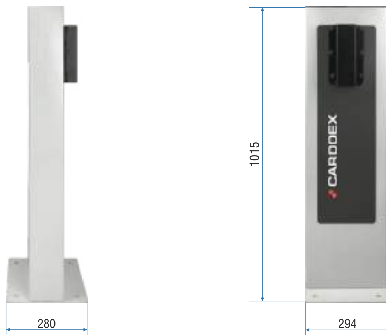
Рисунок 4.1. Габаритные размеры тумбы шлагбаума.
