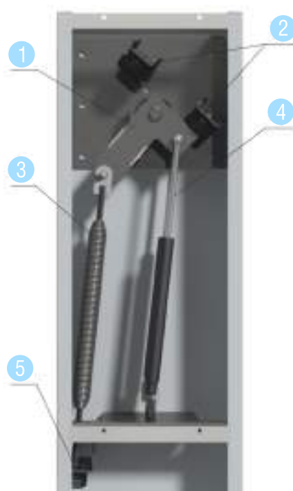
Рисунок 5.1. Устройство шлагбаума.
