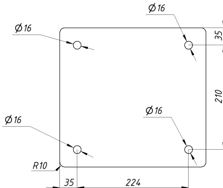
Рисунок 6.4.2. Монтажное основание.
