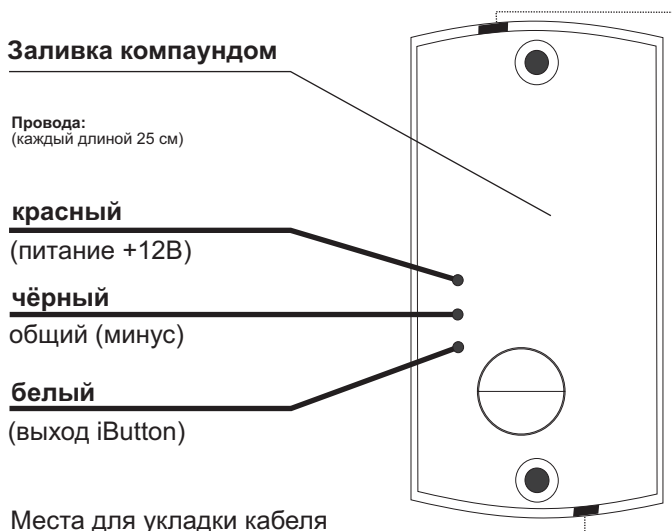
Рис. 3 Вид сзади
