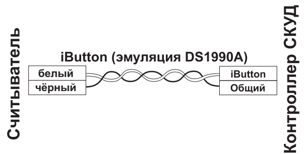
Рис. 4 Схема подключения
