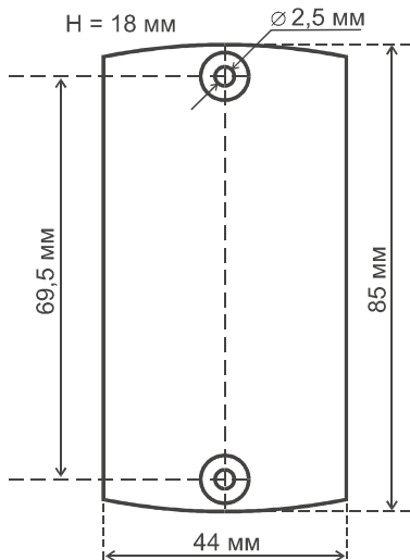
Рис. 1 Габаритные размеры
