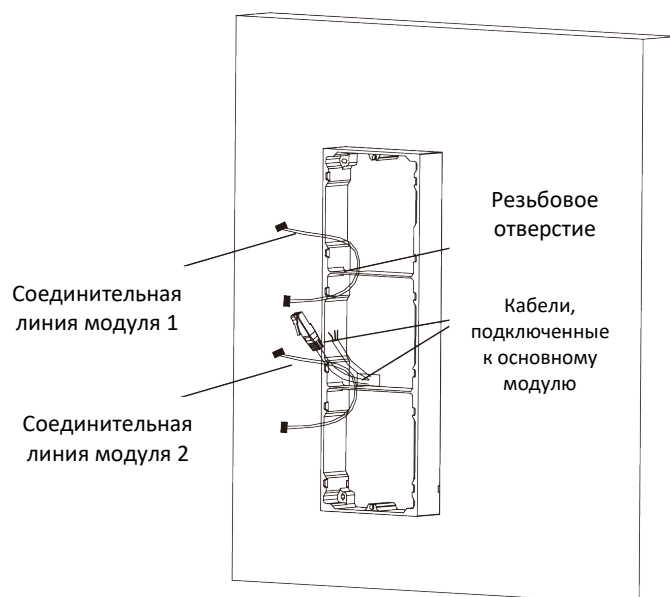
Рисунок 3-33 Размещение линий
