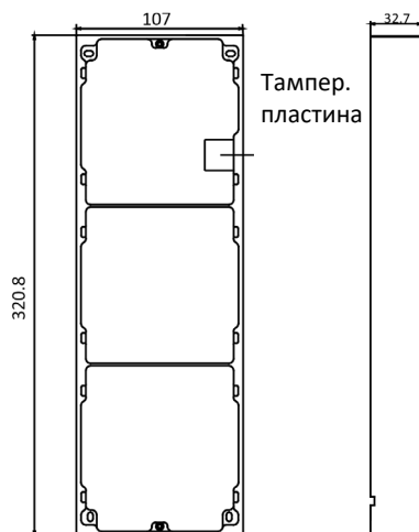
Рисунок 3-44 Монтажная рама
