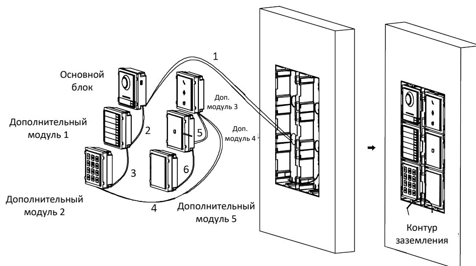
Рисунок 3-60 Установка монтажной рамы
