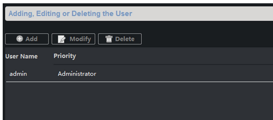
Рисунок 4-6 Страница пользователя
