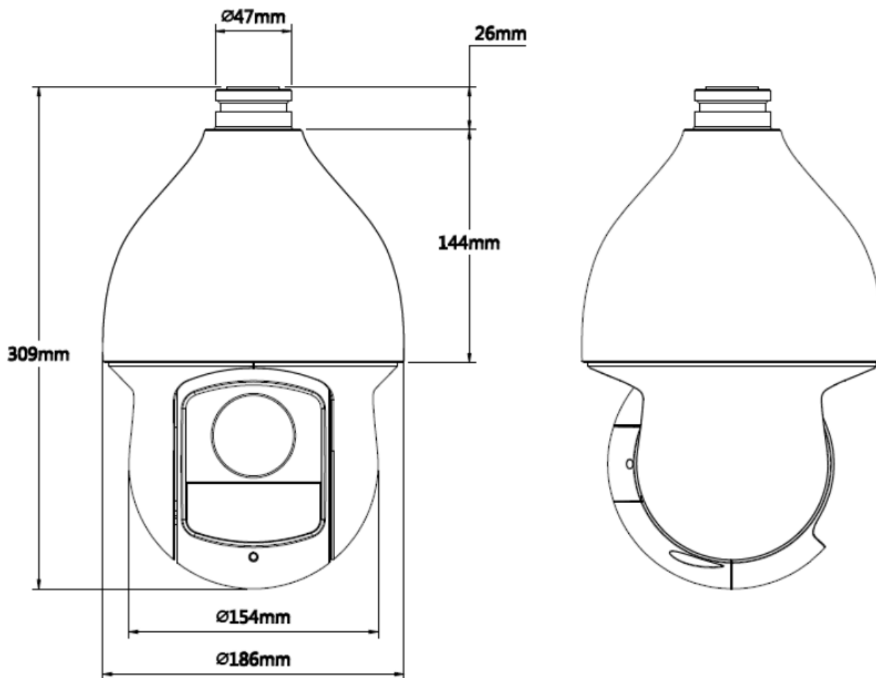
Знешні выгляд камеры ў зборы
