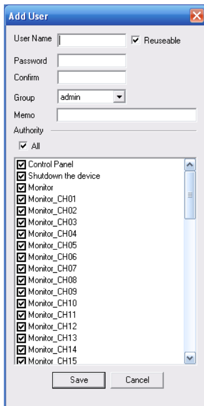
Рисунок 7-51 Добавление пользователя
