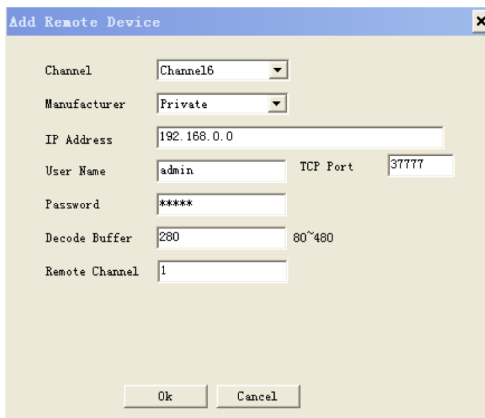
Рисунок 7-55 Добавление вручную
