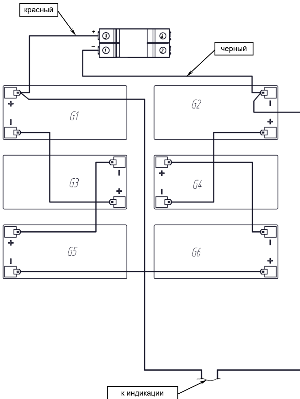
Рисунок 7 — Схема соединений аккумуляторных батарей
