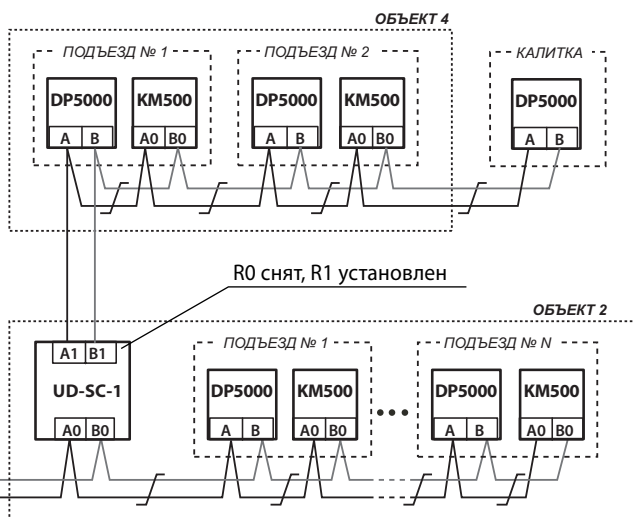
Рис.46 Схема включения разветвителя в СДК сегмент сети из нескольких СУ.
