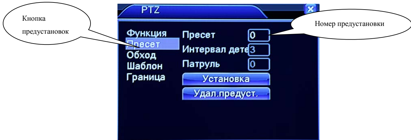
Рис. 3.11 Настройки предустановок
