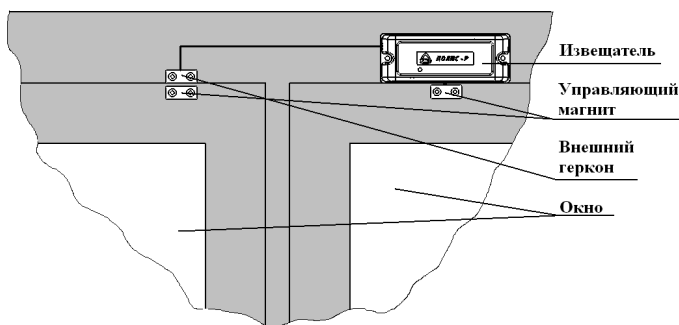
Рис. 8 Размещение на окне
