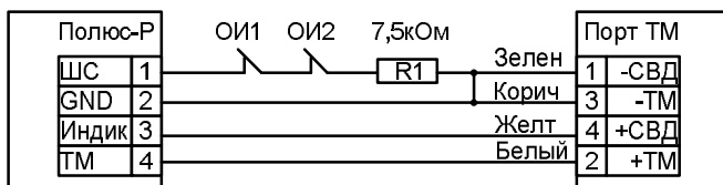
Рис. 14 Подключение шлейфа сигнализации и порта Touch Memory (САПО.425729.001) к извещателю «ПОЛЮС-Р» (ОИ1,ОИ2 – охранные магнитоcontactные извещатели)
