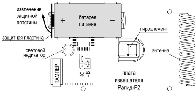
Рис.7 Плата извещателя «Репид-Р2»
