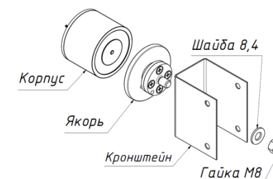
Рисунок 1 - Комплект поставки
