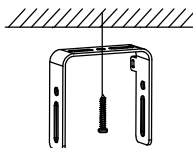
Рисунок 2-3 Установка кронштейна
