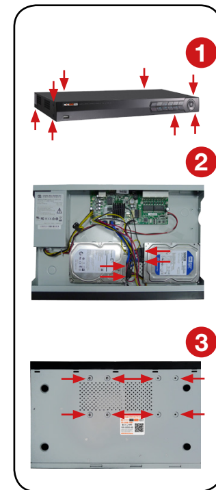
Рисунок 3.3 Установка HDD в IP регистраторах.
