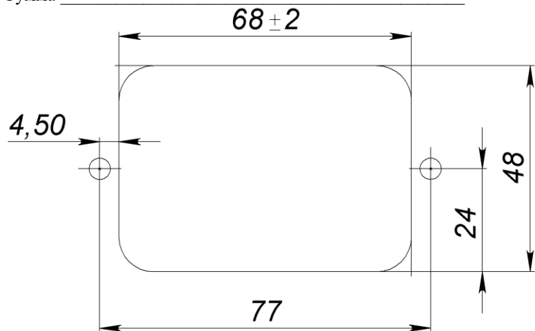
Рис2. Разметка под установку видеокмеры EVM1-IP2-IRM
