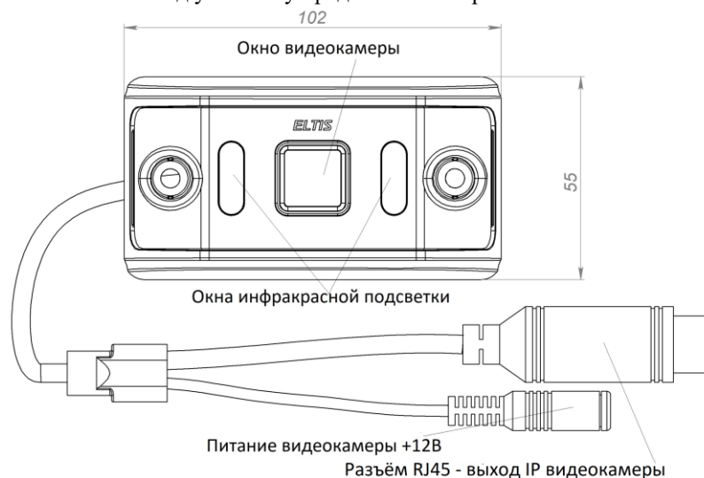
Рис.1 Внешний вид видеокамеры EVM1-IP2-IRM
