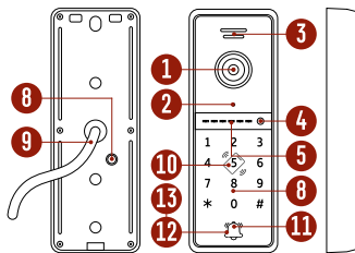
Рис. 4 Вызывная панель FANTASY MRK FHD
