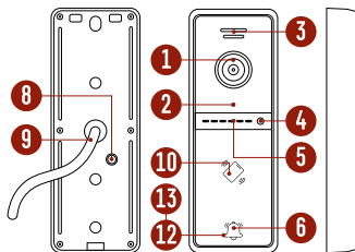
Рис. 3 Вызывная панель FANTASY MR FHD
