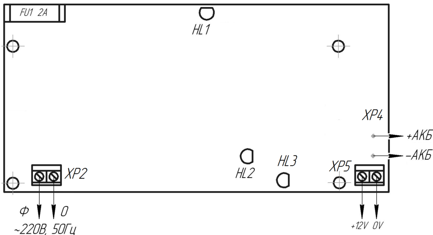
Рис. 1 Схема подключения
