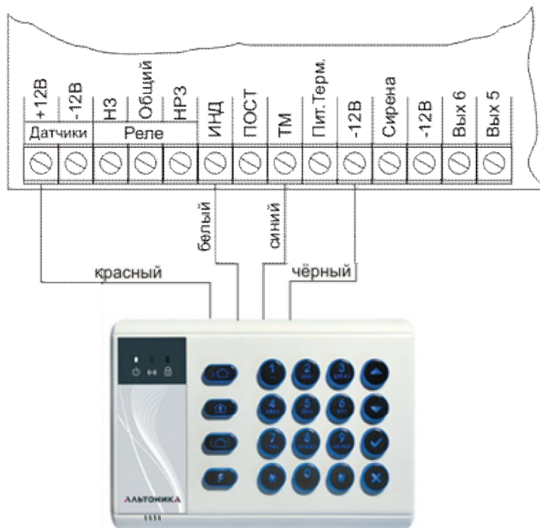
Клемная колодка Часовой 8x8-ВОХ
