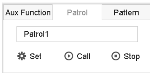
Рисунок 3-14 Настройка патрулирования
