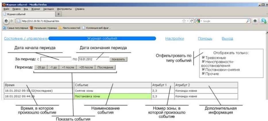
Рисунок 12.8 – Журнал событий
