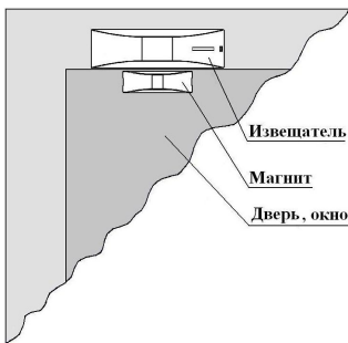
Рисунок 3.9 – Размещение на двери без металлических конструкций
