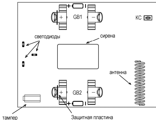
Рисунок 3.13 – Плата «Призма-P2M»
