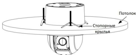
Рисунок 1-21 Врезная установка камеры
