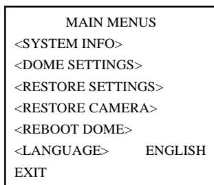
Рисунок 2-2 Главное меню
