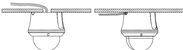
Рисунок 1-23 Прокладка кабелей
