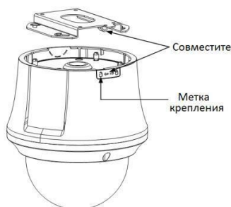
Рисунок 1-27 Накладная установка камеры
