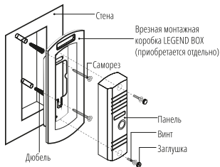
Рис. 7 Врезная установка вызывной панели LEGEND
