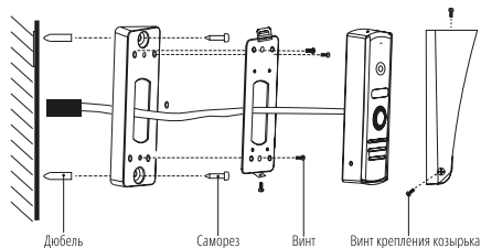
Рис. 9 Установка вызывной панели MASK под углом 30°
