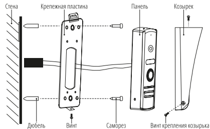
Рис. 8 Фронтальная установка вызывной панели MASK
