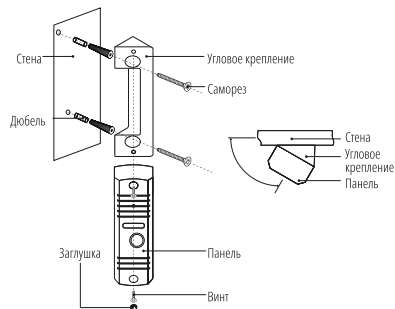
Рис. 6 Установка вызывной панели LEGEND под углом 30°
