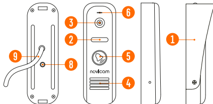
Рис. 3 Вызывная панель MASK
