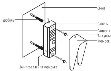
Рис. 5 Фронтальная установка вызывной панели LEGEND
