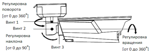
Рисунок 2-16 3-х осевая регулировка
