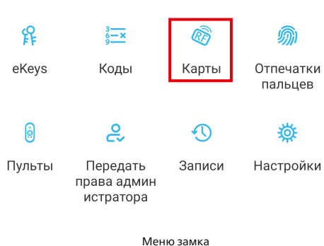
Меню замка
