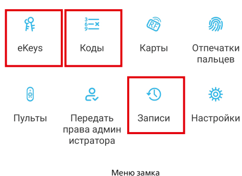
Меню замка
