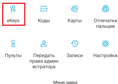
Меню замка
