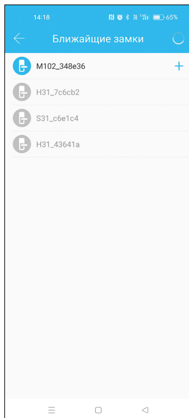
Добавление устройства
