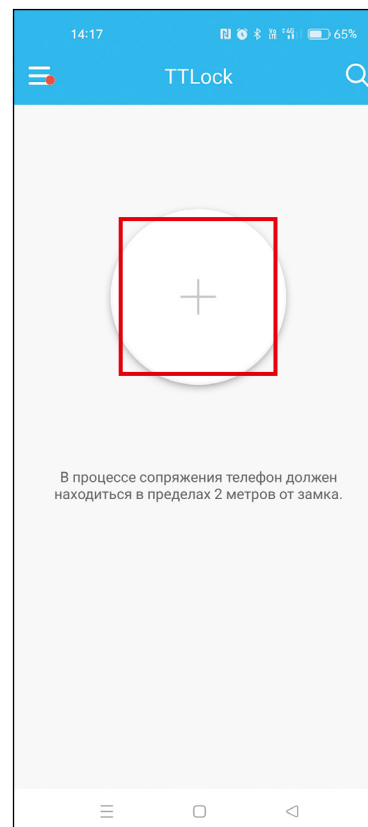
Главный экран
