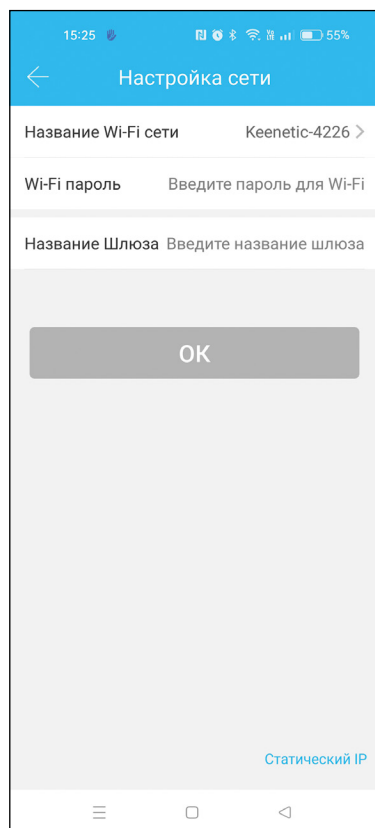
Добавьте "Шлюз"
