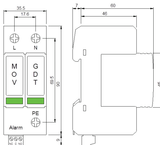
Рис. 1. Внешний вид и габариты TL240L385-1PN
