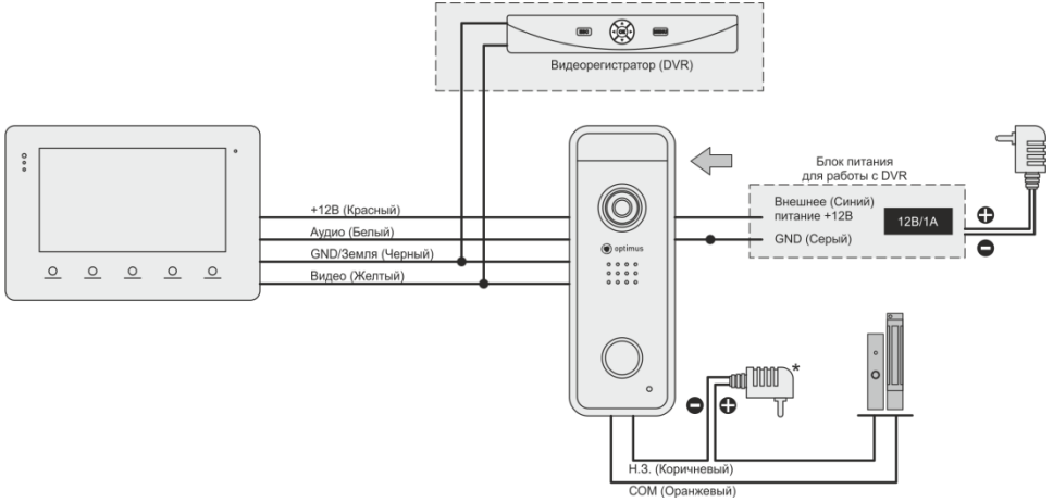
Рисунок 3. Схема подключения №3
