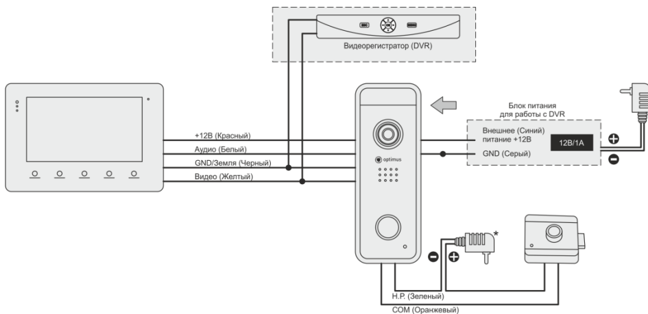
Рисунок 2. Схема подключения №2
