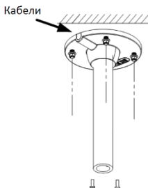
Рисунок 2-39 Установка подвесного кронштейна
