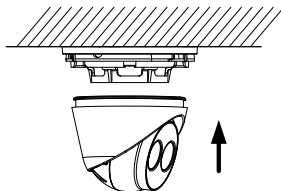
Рисунок 2-27 Установка камеры
