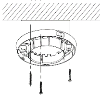
Рисунок 2-33 Установка монтажной платформы
