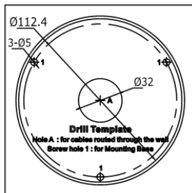
Рисунок 2-2 Шаблон крепления
