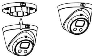
Рисунок 2-34 Установка камеры
