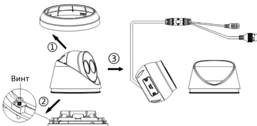
Рисунок 2-23 Демонтаж камеры
