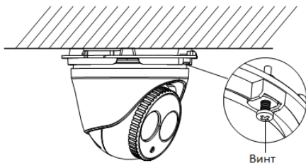
Рисунок 2-6 Фиксирующий винт
