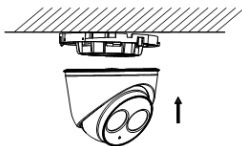
Рисунок 2-20 Установка камеры
