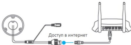
Рисунок 5-3 Подключение к роутеру
