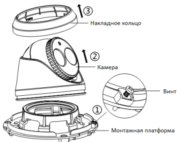
Рисунок 2-1 Демонтаж камеры
