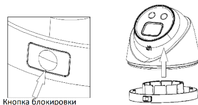
Рисунок 2-30 Демонтаж камеры
