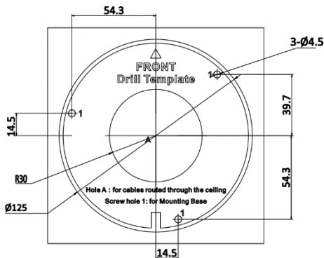
Рисунок 2-32 Шаблон крепления
