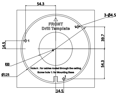
Рисунок 2-25 Шаблон крепления
