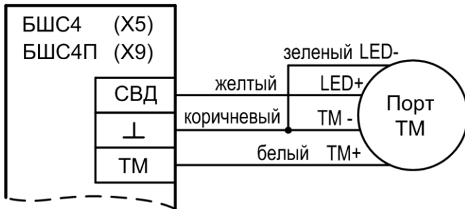
Рис.А12 Схема подключения порта Touch Memory к БШС4 и БШС4П
