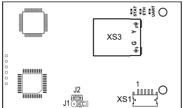
Рис. А18 Внешний вид платы IP-коммуникатора
