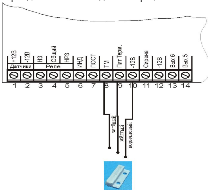
Термодатчик
