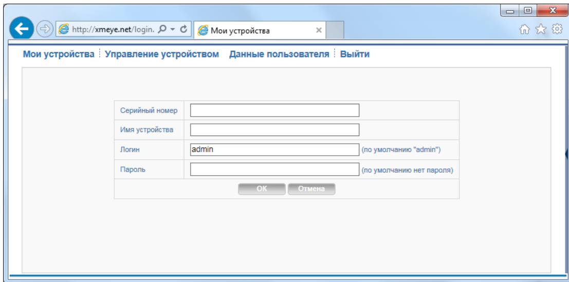
Рис. 5.5 Добавление регистратора
