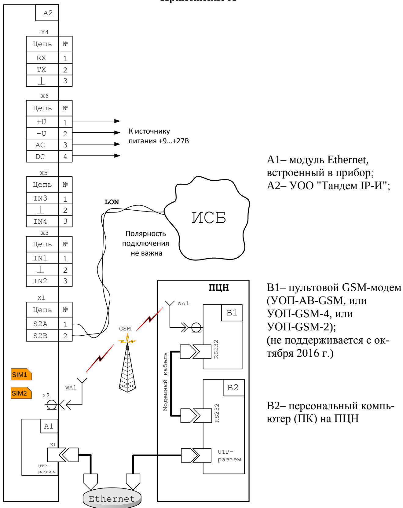
Рисунок А.1 – Схема внешних подключений прибора при работе в составе ИСБ "Стрелец-Интеграл"
