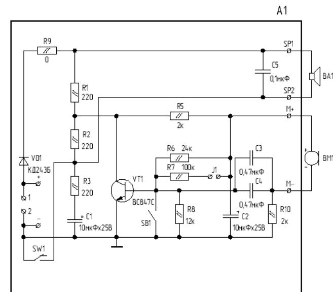
Схема электрическая принципиальная ТАП ЦИФРАЛ КМ-2
