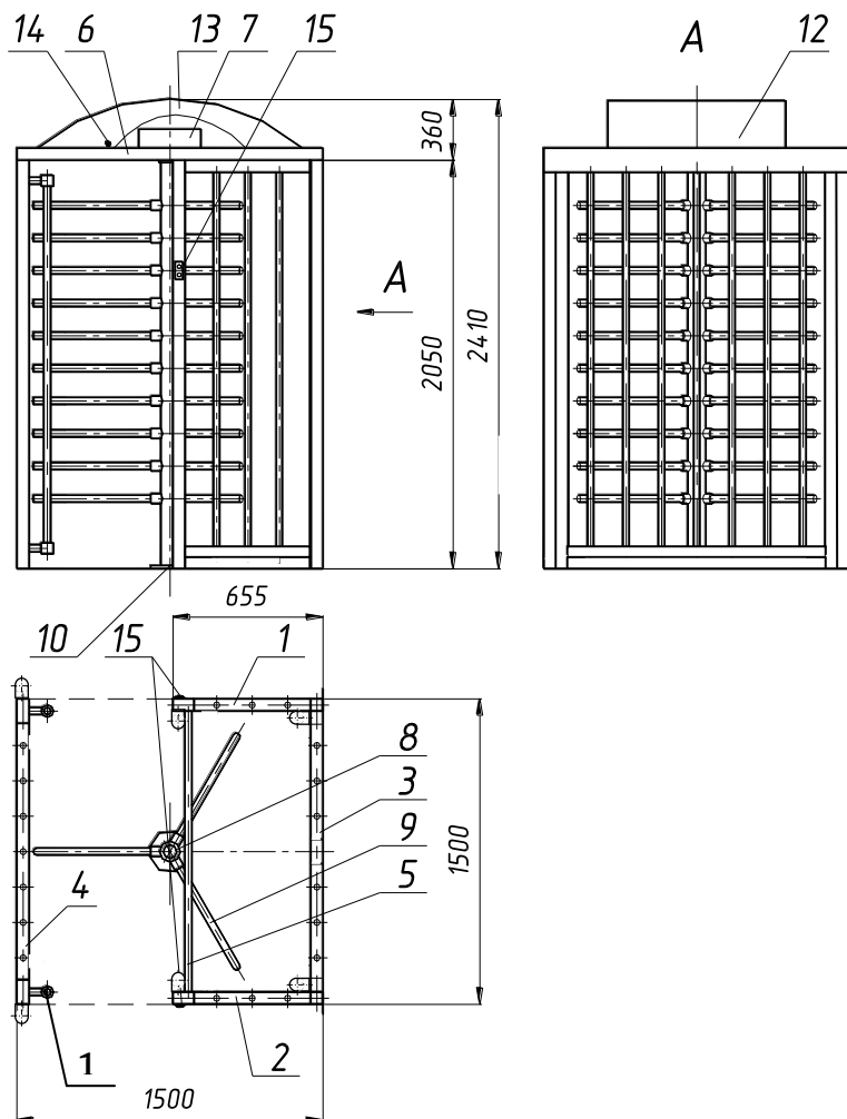
Габаритные размеры турникета «Ростов-Дон ПР1» (поз. 12, 13 – опции)
