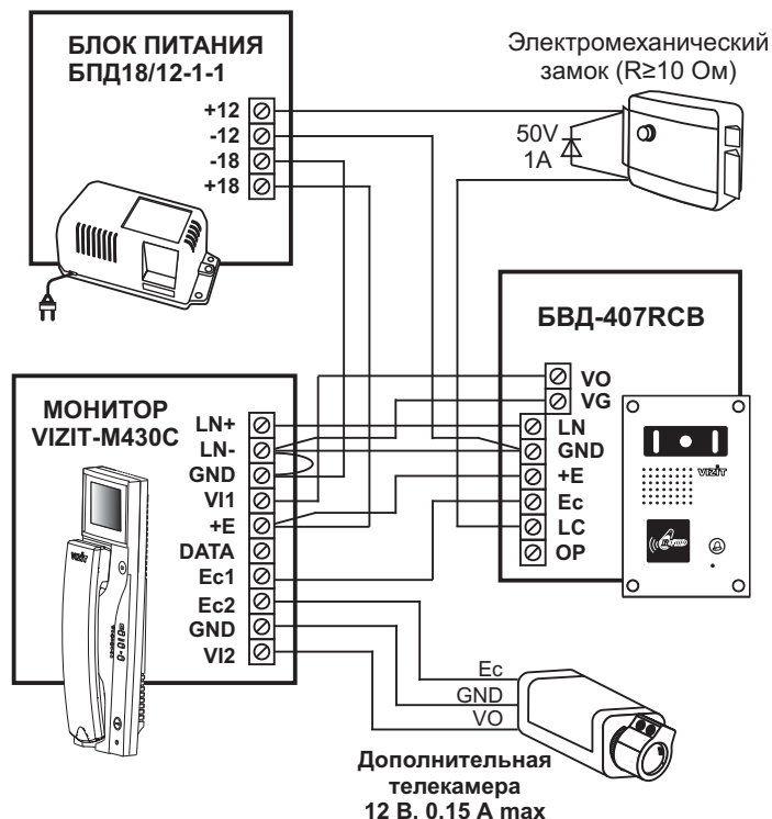
Рисунок 4 - Схема соединений БВД-407RCB с монитором VIZIT-M430C, дополнительной телекамерой и электромеханическим замком
