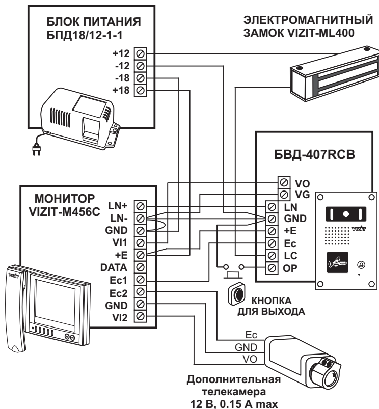
Рисунок 5 - Схема соединений БВД-407RCB с монитором VIZIT-M456C , дополнительной телекамерой и электромагнитным замком
