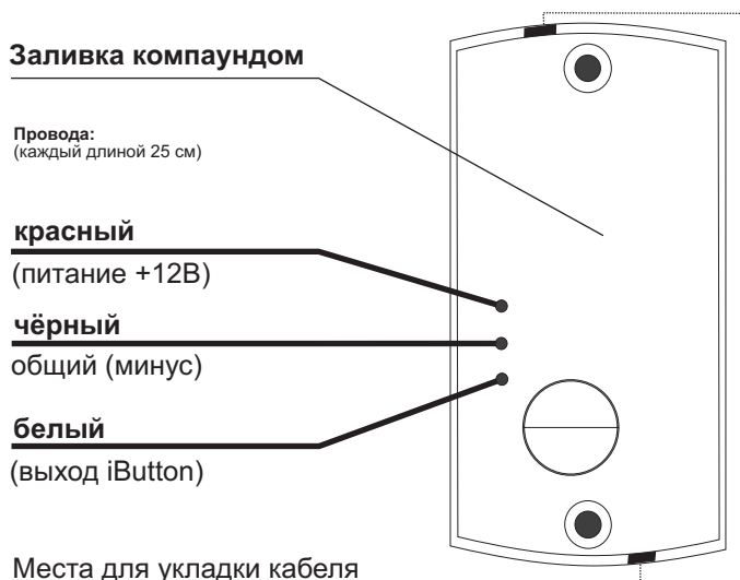
Рис. 3 Вид сзади
