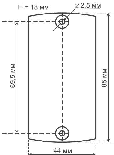
Рис. 1 Габаритные размеры
