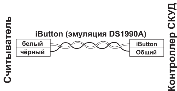
Рис. 4 Схема подключения
