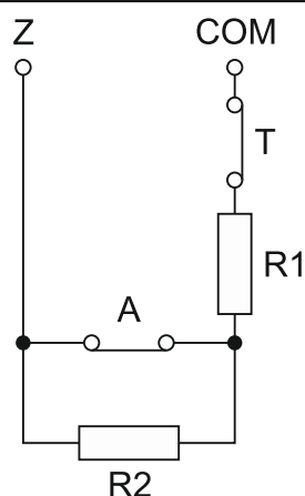
Рис. 4. Нумерация оконечных резисторов. Т – тампер. А – тревога. В случае шлейфов EOL значение резистора – это сумма значений, запрограммированных для резисторов R1 и R2.
