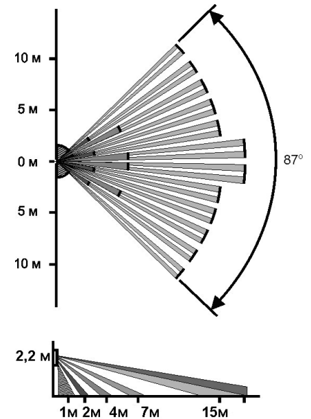
Рис.3 Диаграмма зоны обнаружения при наклоне основания извещателя вперед на угол 12 градусов. Заштрихованная область (антисаботажная зона) только для варианта 2
