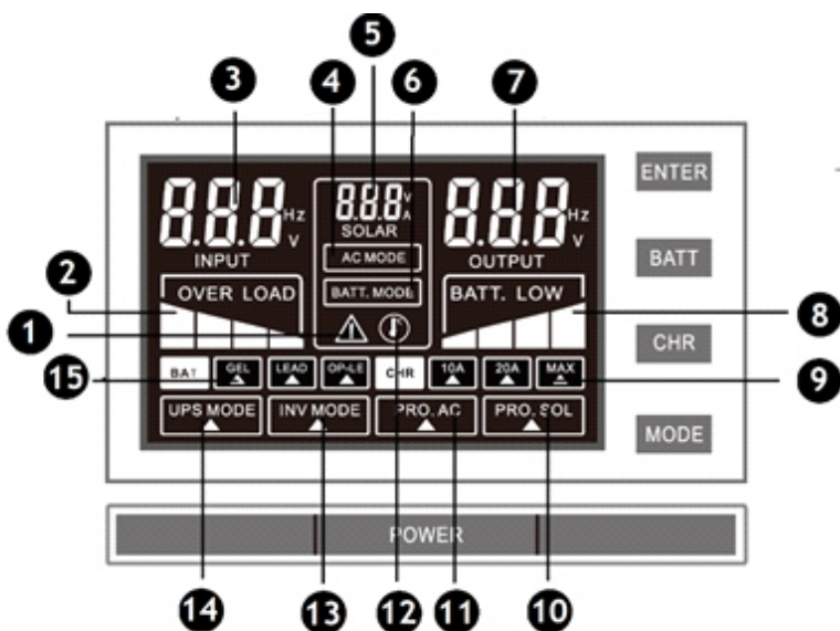
Рис.4 Индикаторы ЖК-дисплея
