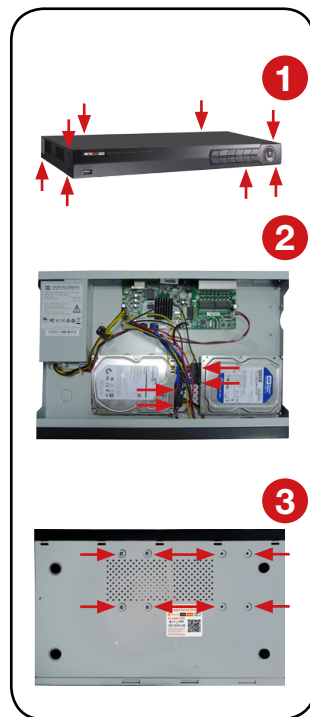
Рисунок 3.2 Установка HDD в IP регистраторах.
