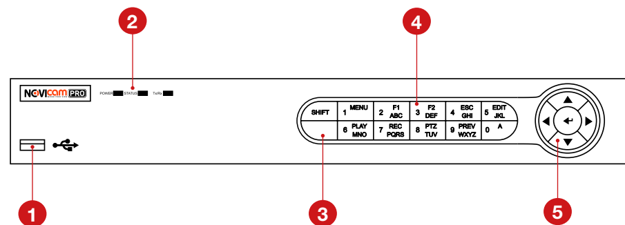
Рисунок 3.7 Передняя панель TVI регистраторов.
