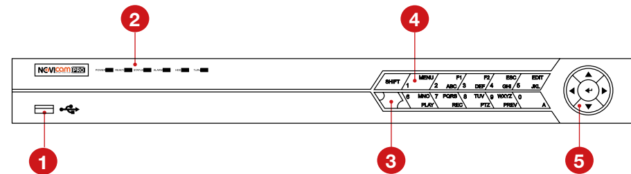
Рисунок 3.5 Передняя панель IP регистраторов (корпус под 2 HDD).
