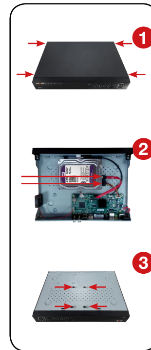
Рисунок 3.3 Установка HDD в TVI регистраторах.
