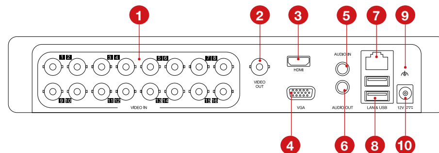
Рисунок 3.8 Передняя панель аналоговых регистраторов.
