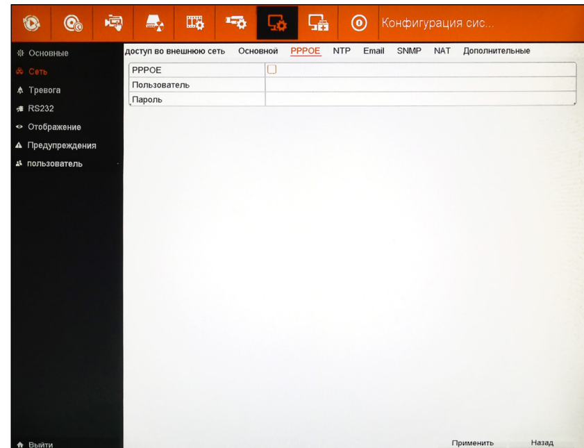
Рисунок 5.71 Настройка PPPOE.
