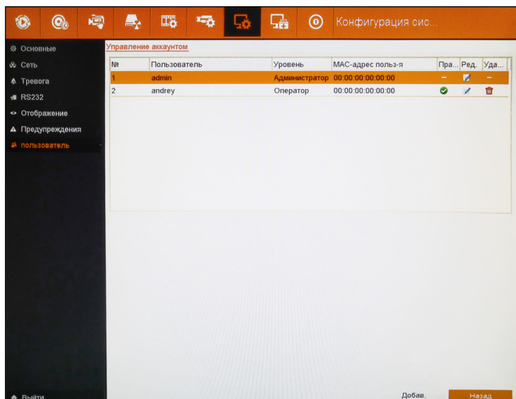
Рисунок 5.92 Окно пользователей.
