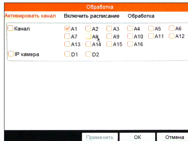
Рисунок 5.56 Выбор каналов.
