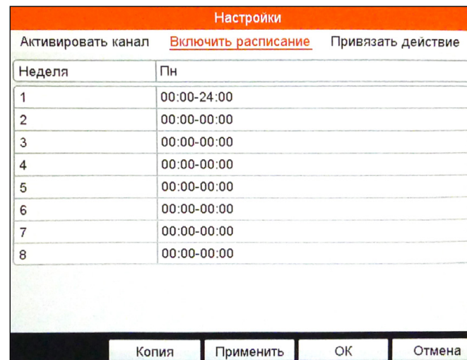
Рисунок 5.57 Установка расписания.
