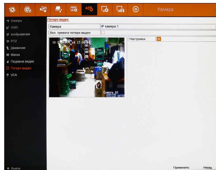
Рисунок 5.61 Потеря видео.
