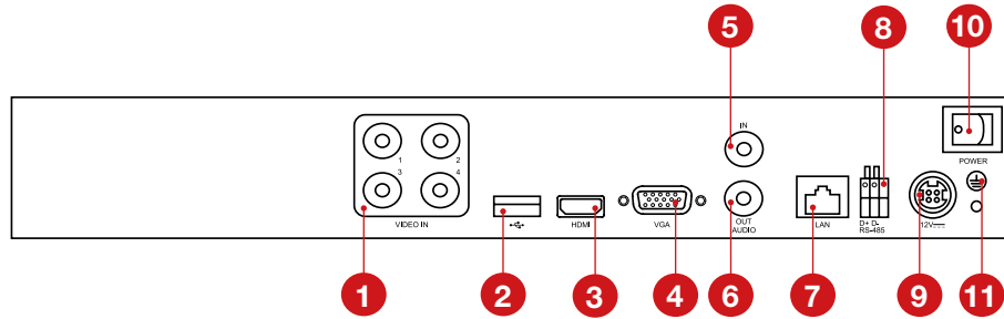
Рисунок 3.13 Задняя панель TVI регистраторов.
