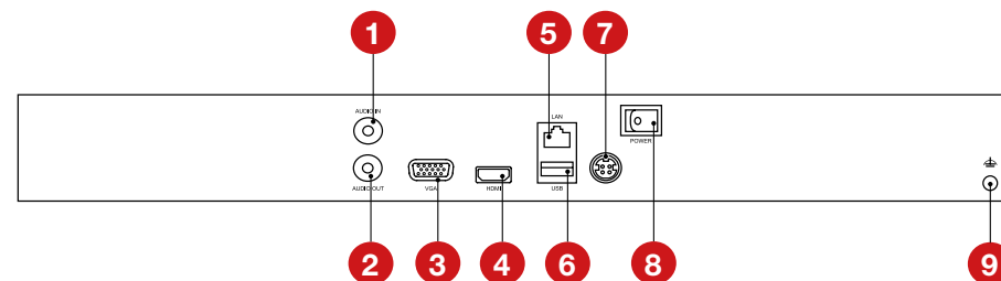
Рисунок 3.10 Задняя панель IP регистраторов (корпус под 2 HDD).
