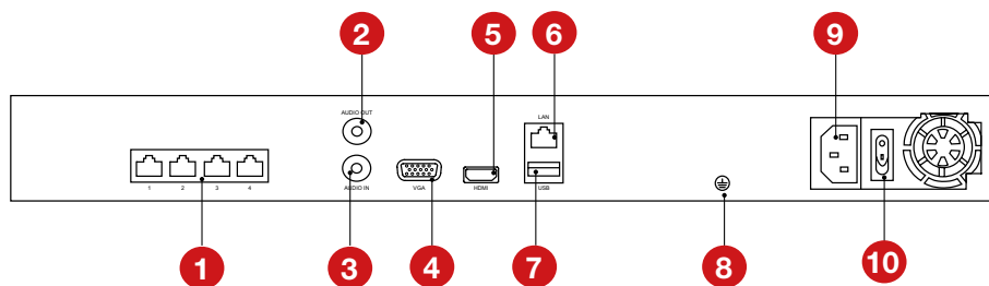
Рисунок 3.9 Задняя панель IP регистраторов (корпус под 2 HDD, 4 PoE).
