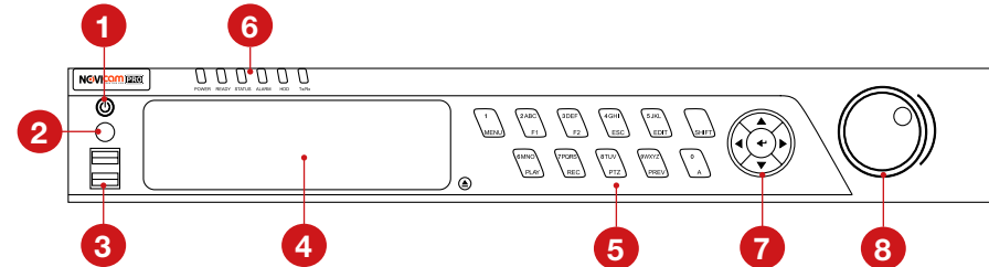
Рисунок 3.6 Передняя панель IP регистраторов (корпус под 4 HDD).
