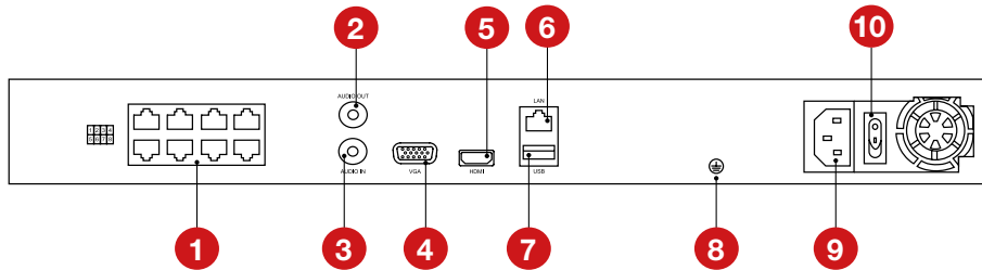
Рисунок 3.11 Задняя панель IP регистраторов (корпус под 2 HDD, 8 PoE).
