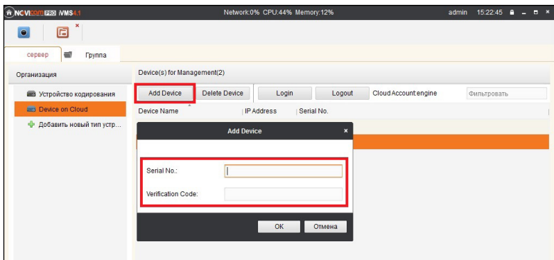
Рисунок 6.13 Добавление устройства.
