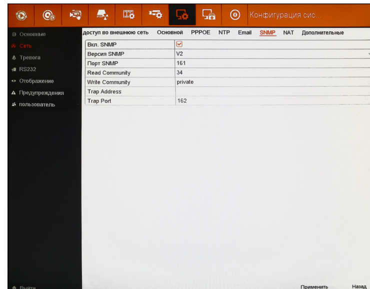
Рисунок 5.77 Настройка SNMP.
