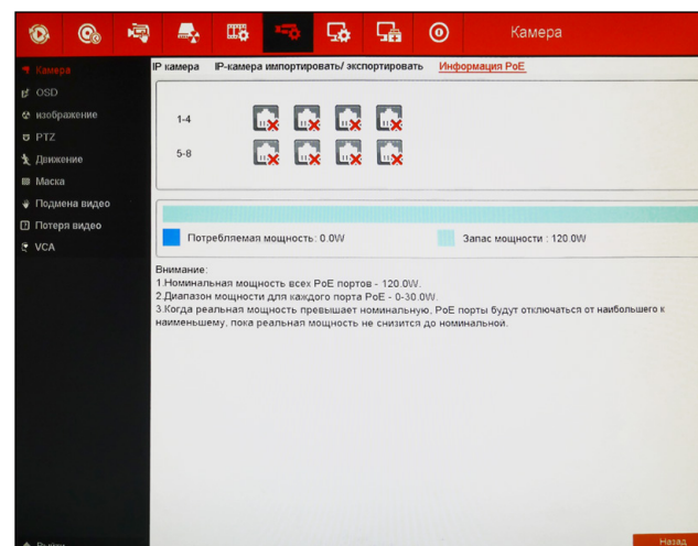
Рисунок 5.48 Информация PoE.
