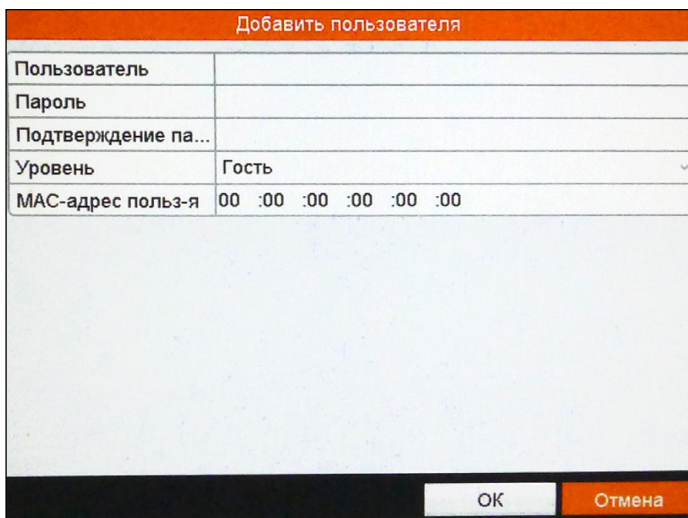
Рисунок 5.93 Добавление пользователя.
