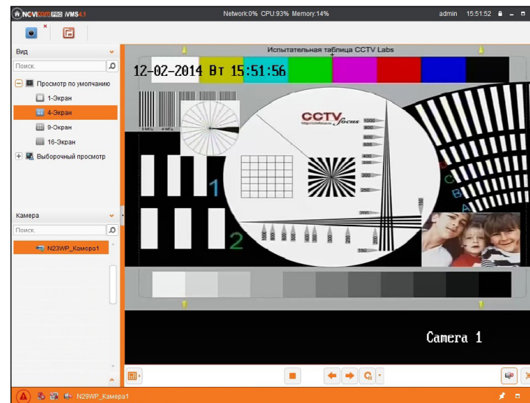
Рисунок 6.18 Просмотр камеры.
