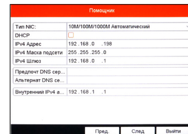
Рисунок 4.5 Настройка сети.
