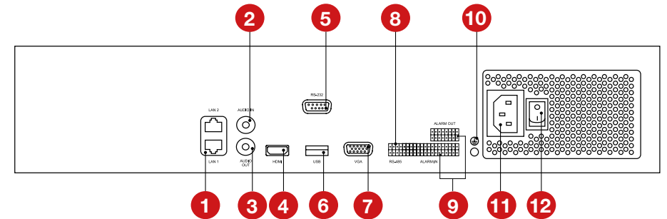
Рисунок 3.12 Задняя панель IP регистраторов (корпус под 4 HDD).
