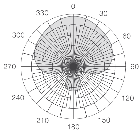
Левая гиперкардиоида
