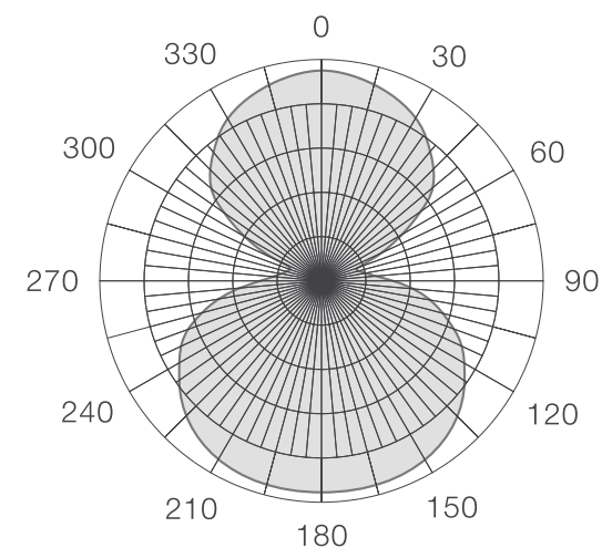
Правая биркардиоида
