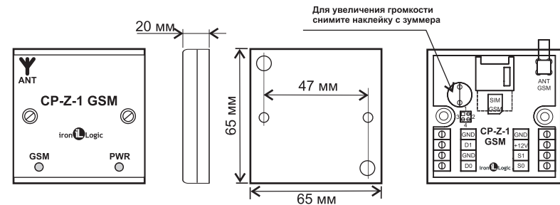
Рис.1 Габариты изделия.
