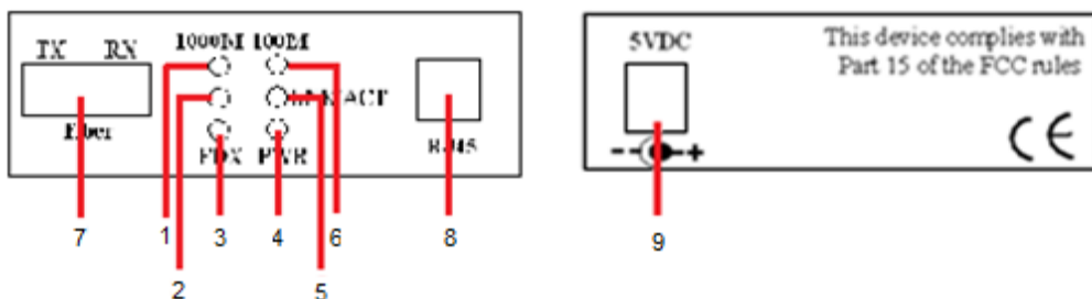
Рис. 3 Элементы медиаконвертеров OMC-1000-11S5a (OMC-1000-11S5b)
