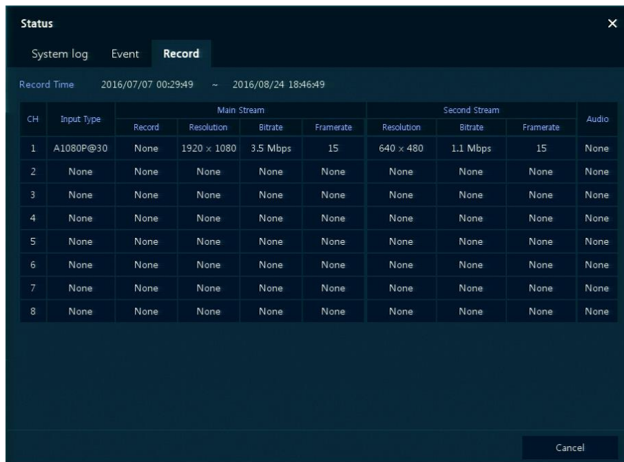
Рис. 3-11 Состояние &gt; Запись в контекстном меню
