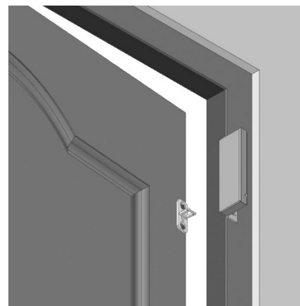
Рисунок 3 - Установка замка на дверь, открывающуюся вовнутрь
