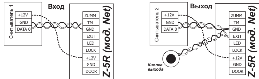
Рис 4. Подключение считывателей.
