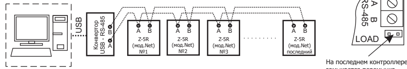
Рис.7 Вариант подключения контроллеров к ПК.
