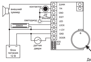
Рис 3. Подключение дополнительных элементов.
