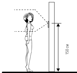
Рис. 7 Рекомендуемая высота установки видеопанели
