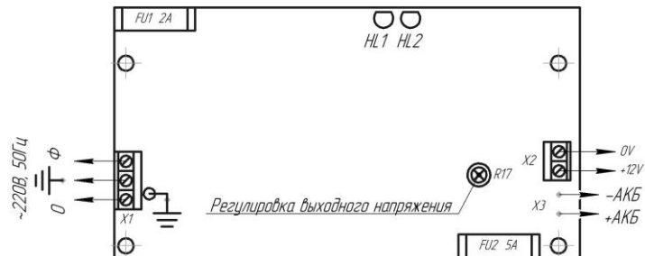
Схема подключения.
