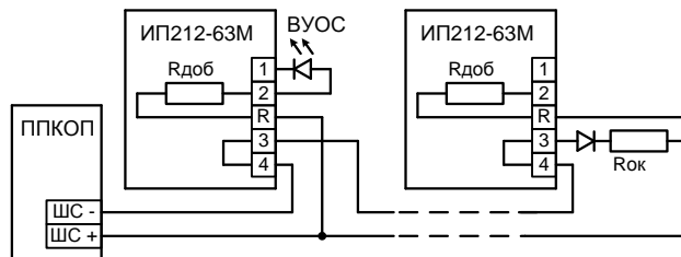
Рис.2 Типовая схема включения извещателя для приборов с переполусовкой шлейфа сигнализации. Величина резисторов Rok и Rдоб определяется в соответствии с техническим описанием ППКОП
