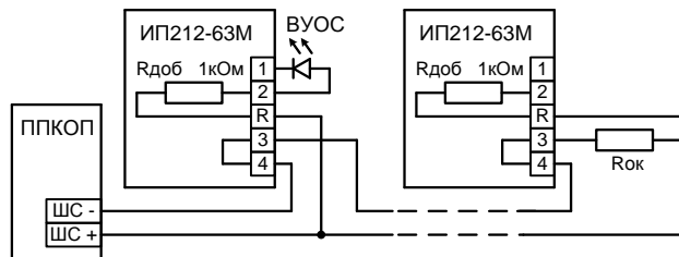
Рис.1 Типовая схема включения извещателя для приборов с однополярным шлейфом сигнализации. Величина резистора Rok определяется в соответствии с техническим описанием ППКОП
